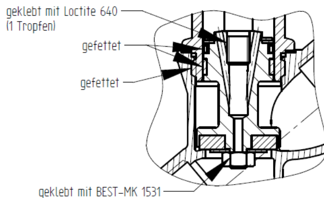
Funktion druckentlastet
